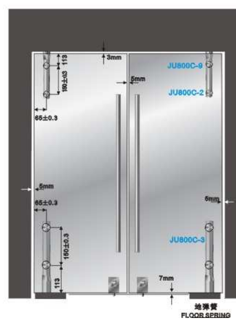
● 安装示例F INSTALLING F
