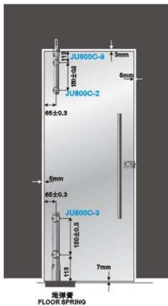
● 安装示例B INSTALLING B
