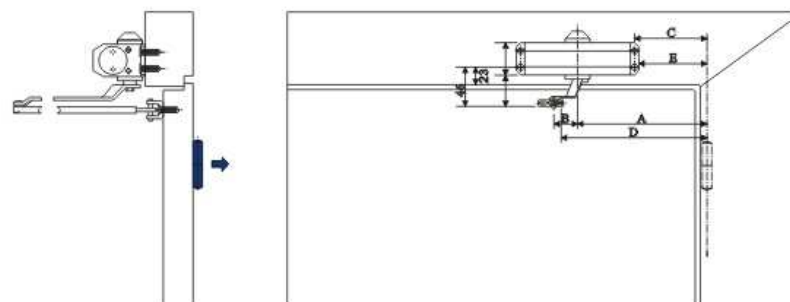
门框安装
