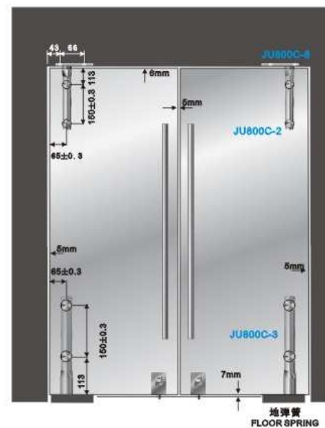
● 安装示例F INSTALLING F
