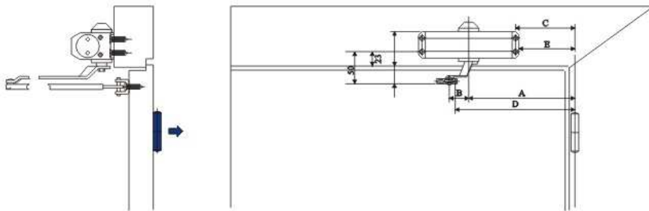
门框安装
