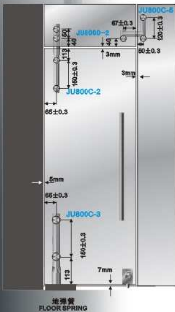
● 安装示例A INSTALLING A
