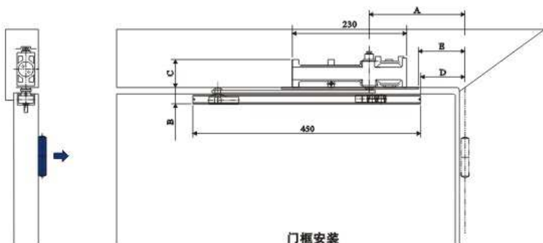
门框安装
