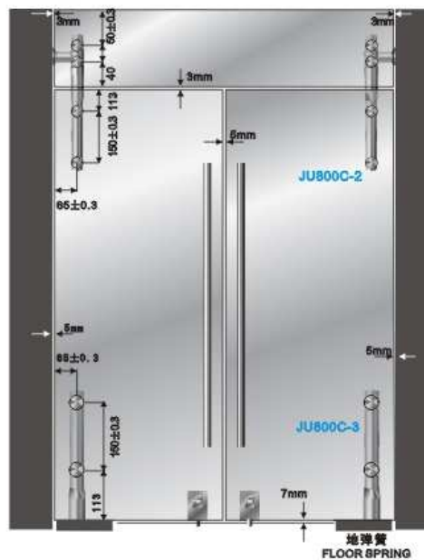
● 安装示例E INSTALLING E
