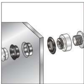
● JU800F-2 玻璃与墙体固定件 Single point fixing (可调节, 调节节位2.5至11.5mm) Adjustable, adjusted 2.5mm—11.5mm
