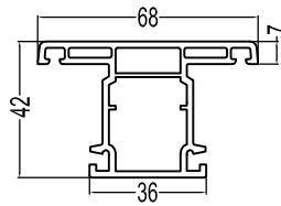
42Sash Mullion P42MSZT 0.72kg/m
