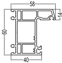
60Casement Frame(A) P60K(A) 0.87kg/m
