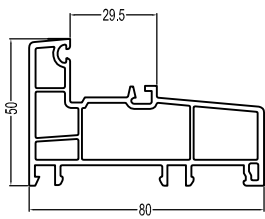
80Upper Sliding Frame(D) T80LK(D) 1.01kg/m
