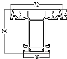
60Casement Mullion(E) P60ZT(E) 1.03kg/m
