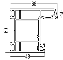
60Casement Frame(C) P60K(C) 0.99kg/m
