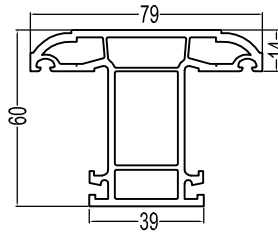
60Casement Mullion(LA) P60ZT(LA) 1.12kg/m
