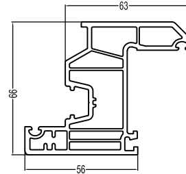
66Inswing Sash(D) P66NKCS(D) 1.35kg/m
