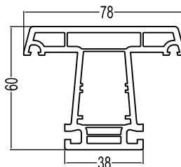
60Casement Mullion(S) P60ZT(s) 1.32kg/m
