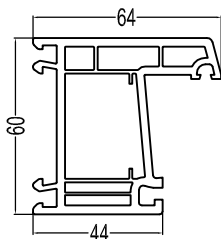
60Casement Frame(S) P60K(s) 1.25kg/m
