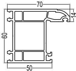
60Casement Frame(LA) P60K(LA) 1.1kg/m
