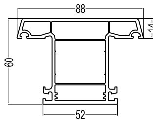
60Casement Mullion(D) P60ZT(D) 1.2kg/m
