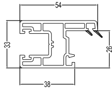
75Sliding Sash T75S 0.67kg/m
