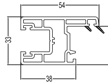
75Sliding Sash(B) T75S(B) 0.62kg/m
