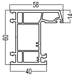
60Casement Frame(B) P60K(B) 1.08kg/m
