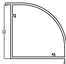
60Corner Profile(90) 60ZJ(90) 0.62kg/m
