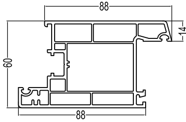
60Casement Inward Door (A) P60NKMS (A) 1.38kg/m
