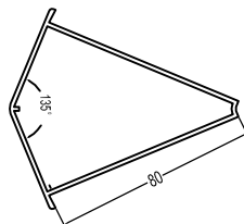
135Corner Profile(80) 135ZJ(80) 0.68kg/m
