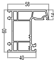
60Casement Frame(E) P60K(E) 0.98kg/m
