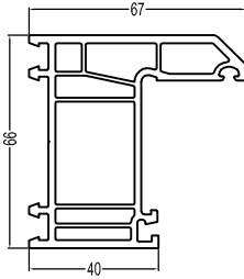
66Casement Frame(D) P66K(D) 1.2kg/m
