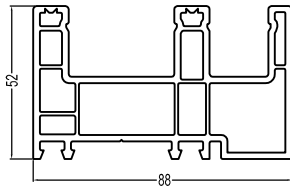
88 Sliding Frame (A) T88K (A) 1.4kg/m
