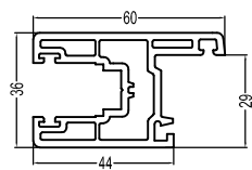
80Sliding Sash(D) T80S(D) 0.82kg/m
