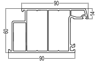
60Casement Door Sash P60MS 1.3kg/m
