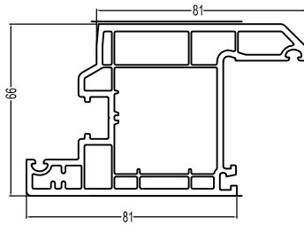
66Casement Inward Door(D) P66NKMS(D) 1.7kg/m
