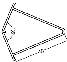
135Corner Profile(60/66) 135ZJ(60/66) 0.52kg/m
