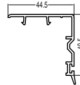
60Weather Strip(B) T60FG(B) 0.26kg/m
