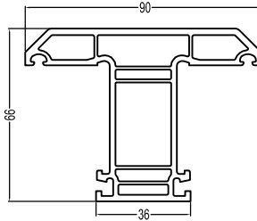
66Casement Mullion(D) P66ZT(D) 1.31kg/m
