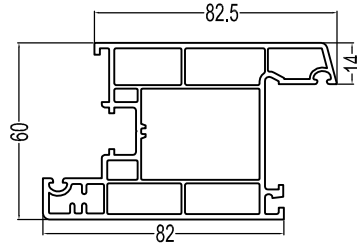
60Casement Inward Door (B) P60NKMS (B) 1.2kg/m
