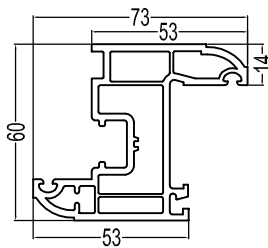
60Inswing Sash(LB) P60NKCS(LB) 1.14kg/m
