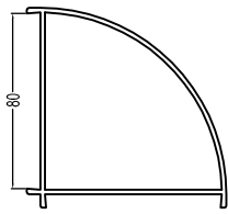
80Corner Profile(90) 80ZJ(90) 0.9kg/m
