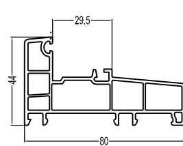
80Upper Sliding Frame(B) T80LK(B) 0.82kg/m
