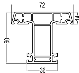
60Casement Mullion(A) P60ZT(A) 0.89kg/m
