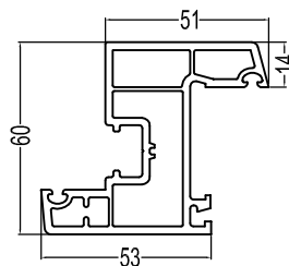
60Inswing Sash(B) P60NKCS(B) 1.12kg/m
