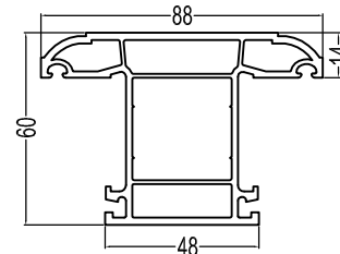
60Casement Mullion(LB) P60ZT(LB) 1.2kg/m
