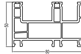
80Sliding Frame(D) T80K(D) 1.22kg/m
