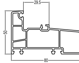
80Upper Sliding Frame(C) T80LK(C) 0.9kg/m
