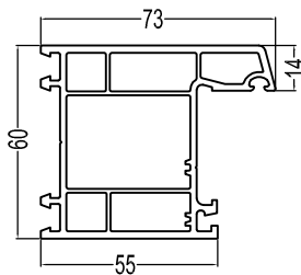
60Casement Frame(D) P60K(D) 1.14kg/m
