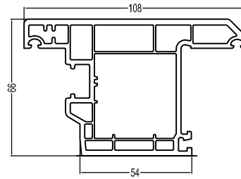
66Casement Outward Door(D) P66WKMS(D) 1.7kg/m
