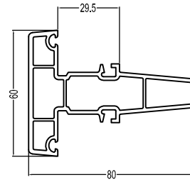
80Upper Sliding Transom(D) T80LT(D) 1.02kg/m
