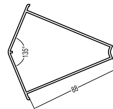
135Corner Profile(88) 135ZJ(88) 0.68kg/m
