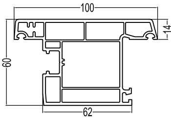
60Casement Outward Door P60WKMS 1.38kg/m
